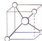
Fig. 4.10 Estrutura tetraédrica.
