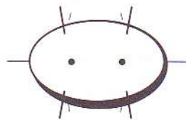
Fig. 4.2 Representação simplificada para o orbital molecular do H_2 .
