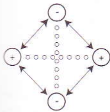
Fig. 4.1 Forças electrostáticas na molécula H_2 .
